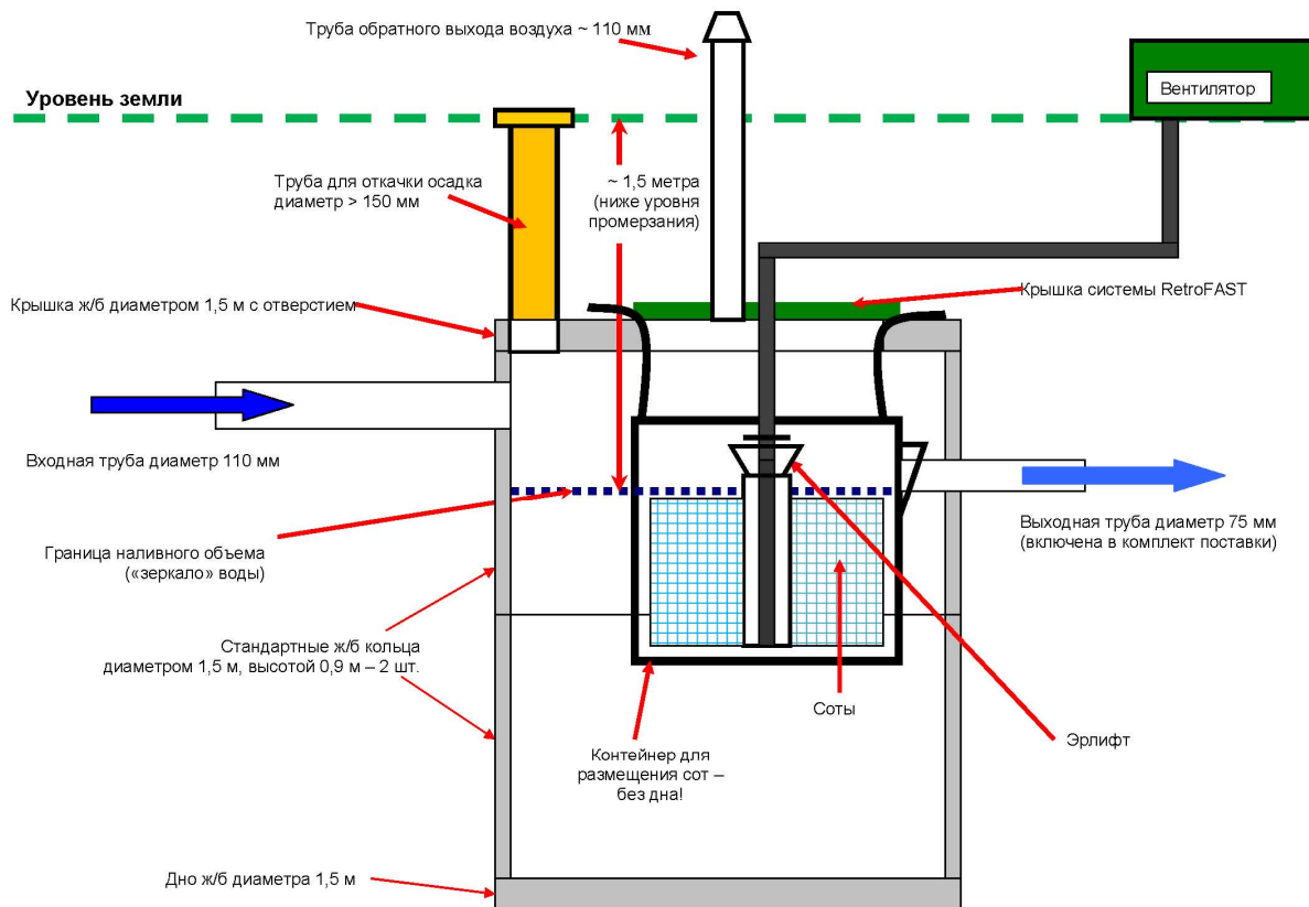
Рис.1. Технологический процесс очистки.
